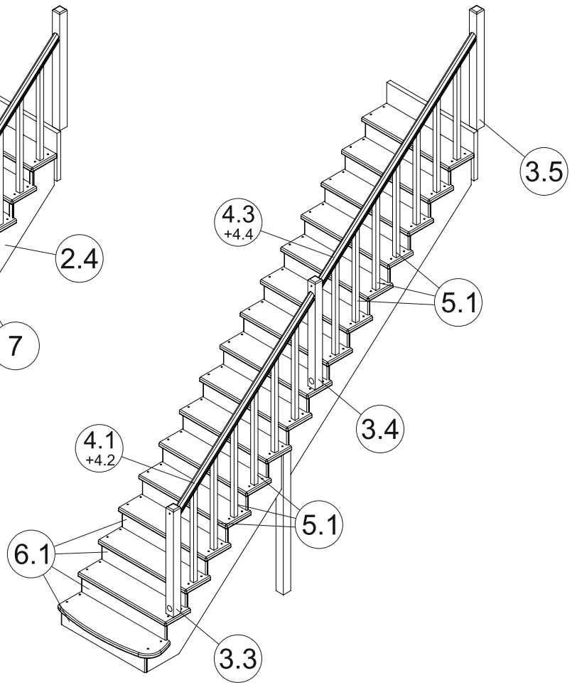
С подступенниками
